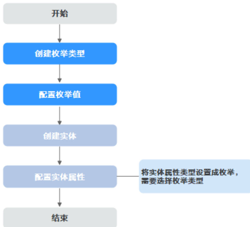
图 5-10 枚举类型配置使用流程
