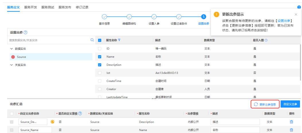
图 9-22 更新提示
