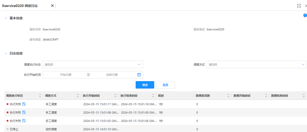
图 9-19 调度日志
