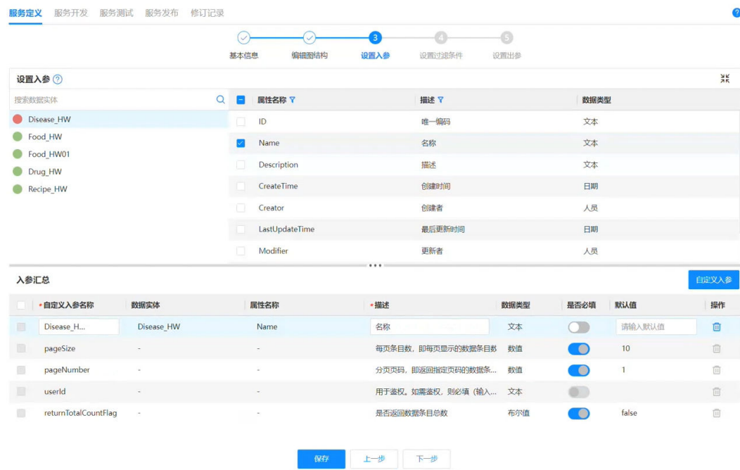
图 9-7 设置入参
