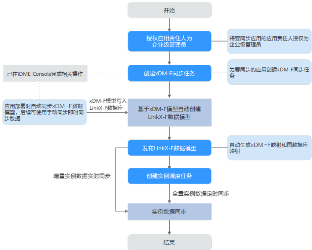
图 4-2 xDM-F 数据同步推荐业务流程二
